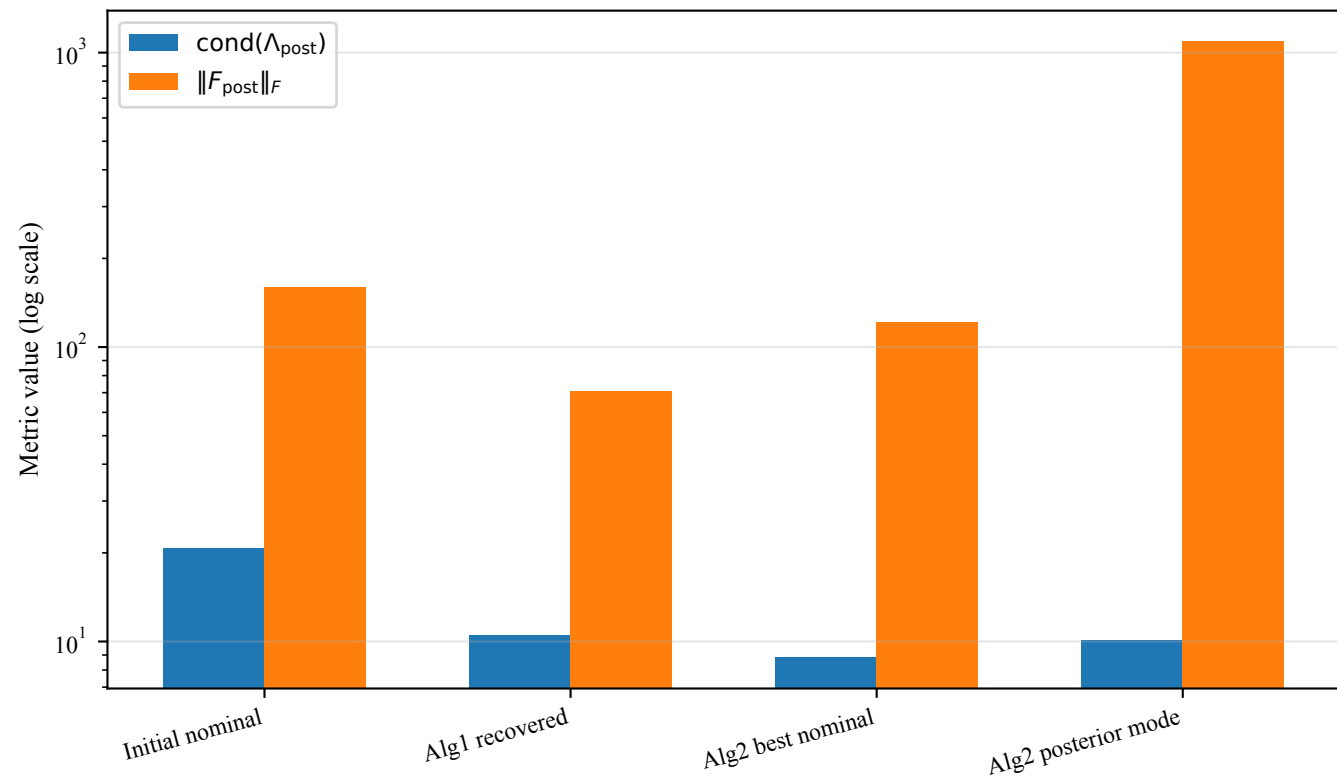
Posterior health metrics
